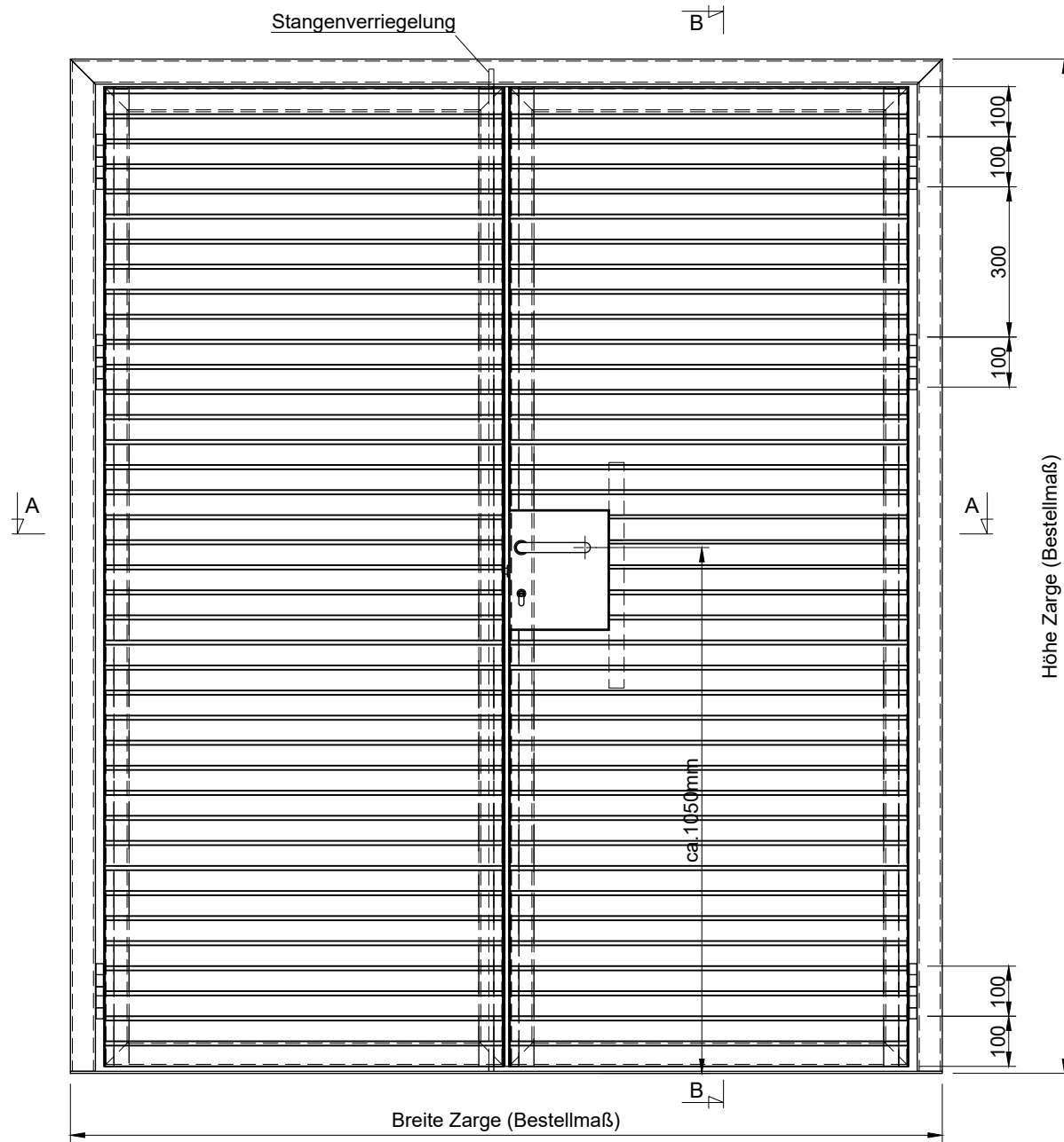
Vorderansicht
