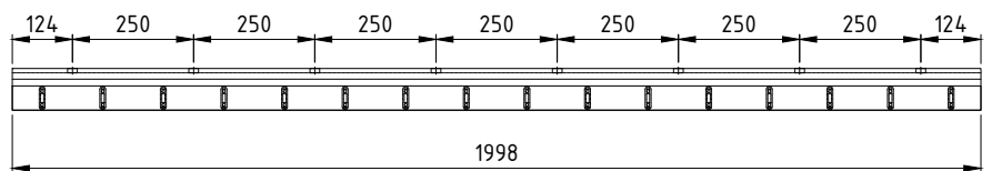
Draufsicht: "B" - Geländerstab abgerundet
